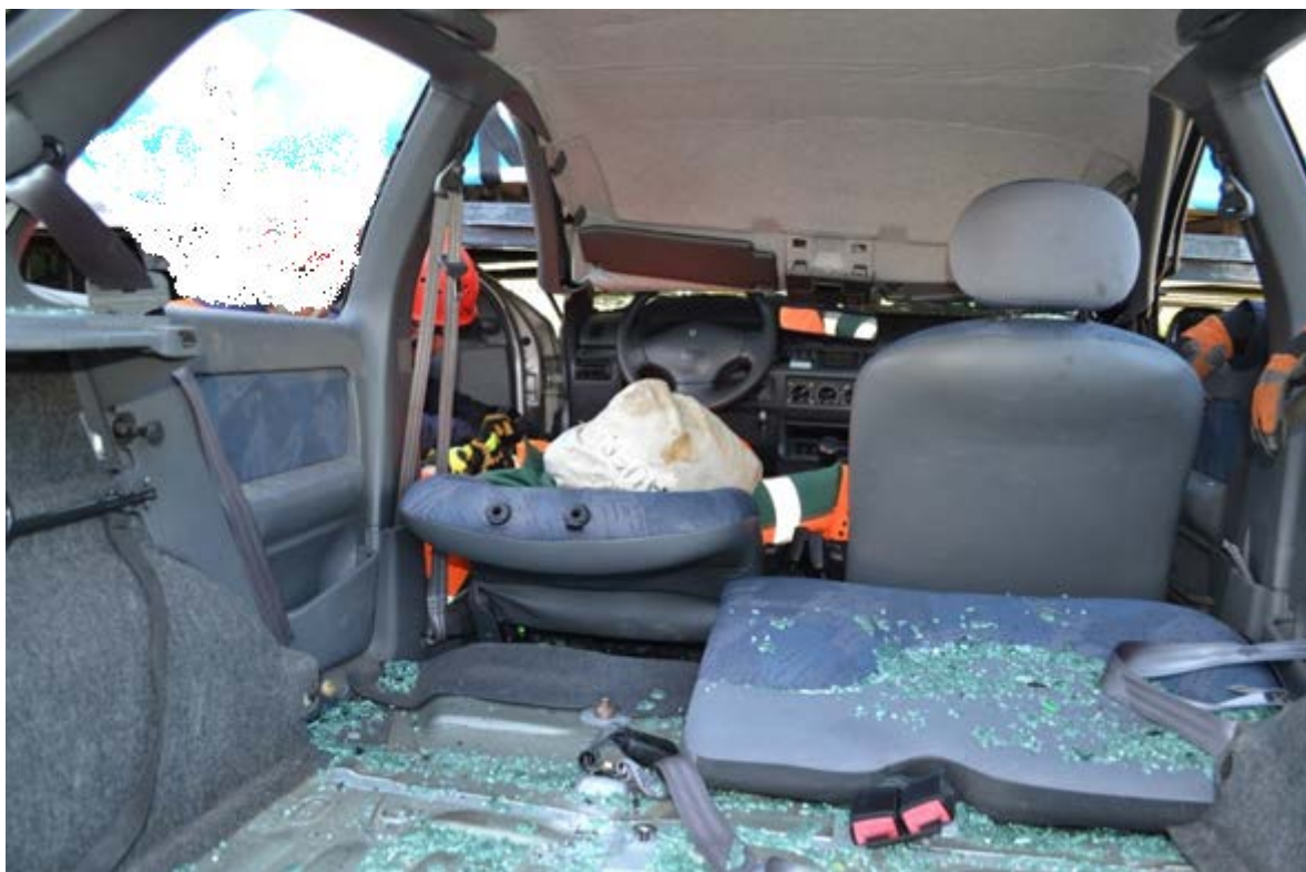
Rys. 356. Szeroki dostęp do osoby poszkodowanej, po wykonaniu techniki „tunelowania”
