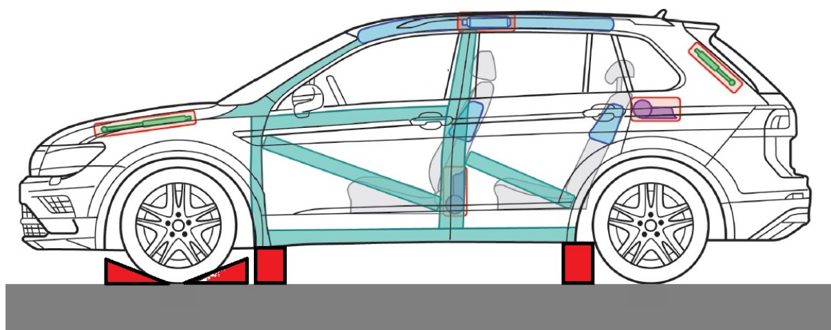
Rys. 158. Stabilizacja czteropunktowa z jednoczesnym zabezpieczeniem przed toczeniem za pomocą klinowania na jednym kole – widok z boku
