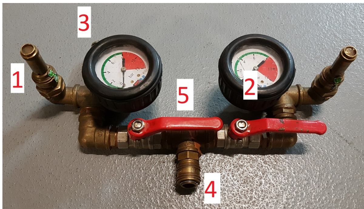
1. Zawór bezpieczeństwa. 2. Wskaźniki ciśnienia (manometr). 3. Szybkozłęczka wyjściowa. 4. Szybkozłęczka wejściowa. 5. Urządzenie sterujące
