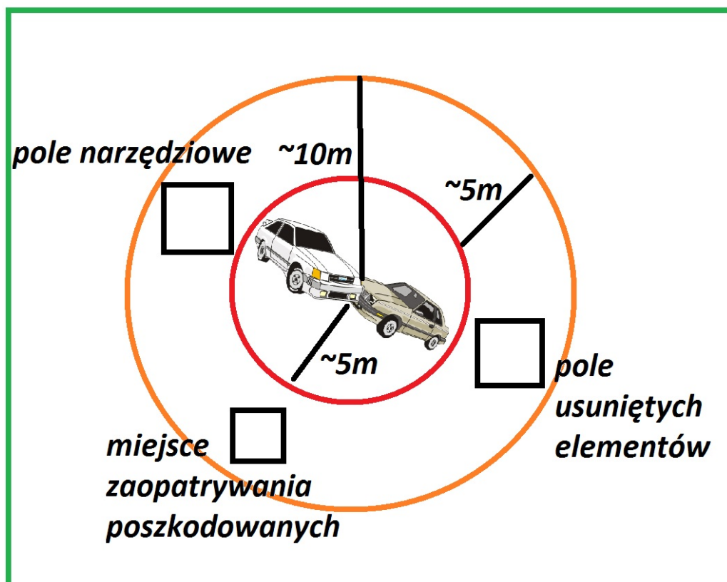
Rys. 123. Schemat podziału terenu akcji ratowniczej
