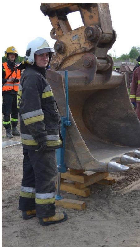
Rys. 390. Podbudowa łyżki drewnem
