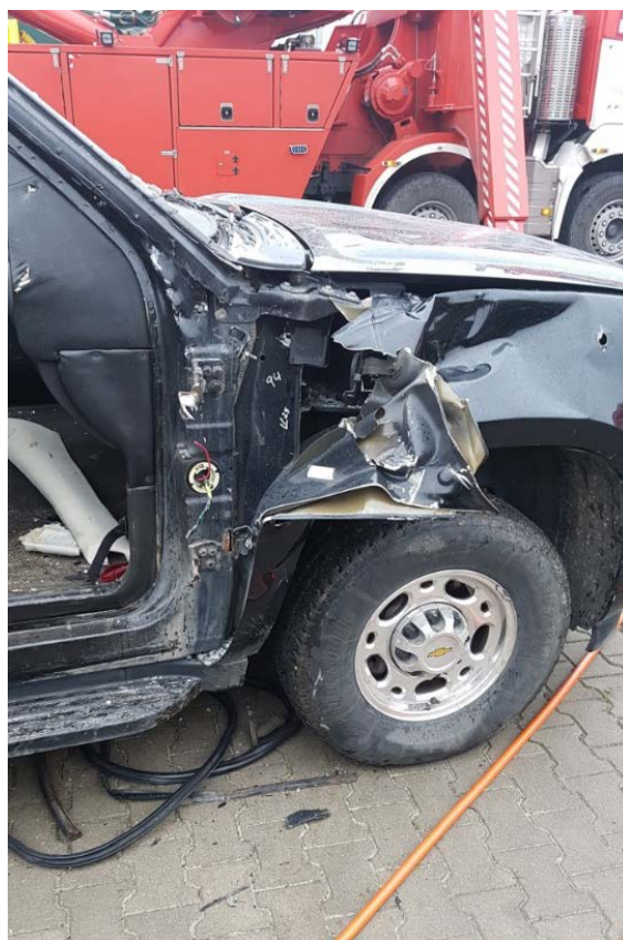
Rys. 132. Nadkole po odgięciu, celem rozpoznania sytuacji pod spodem
